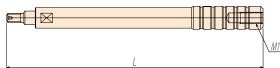
プルボルト取り外し用延長 Bar Extension bar for installing and removing pull bolt
